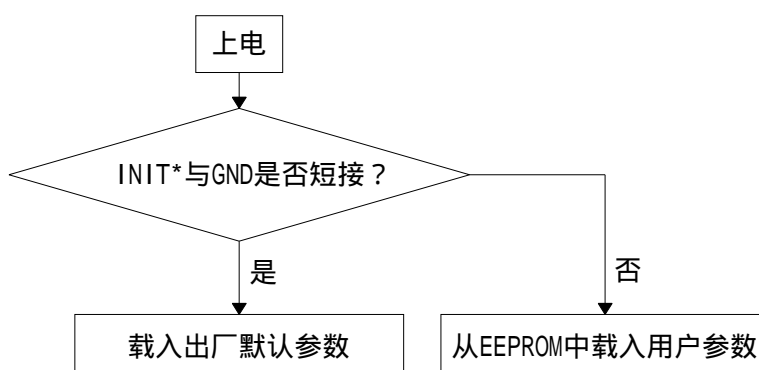
图2.6.2 IR-2033 启动过程及参数载入流程图
