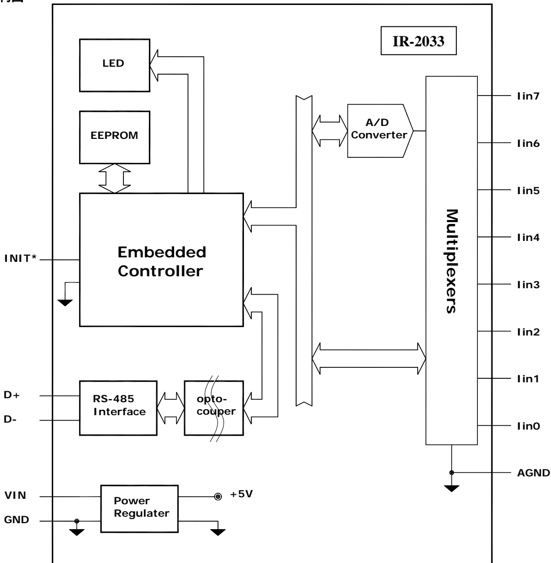
图1.5 IR-2033内部结构框图
