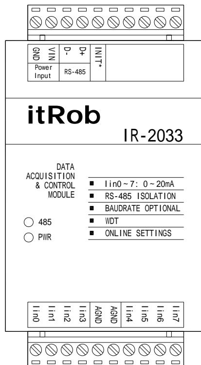
图1.3 IR-2033端子分布
