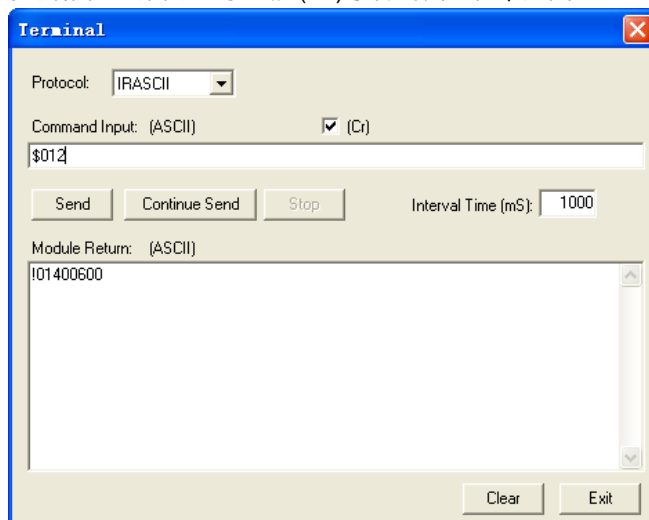
图2.2.6.a (IRASCII协议时的命令与返回信息)
