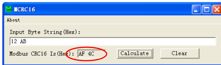
图F.1 MCRC16的计算结果
