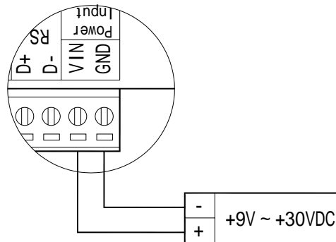
图2.1.5 IR-2033的电源接线
